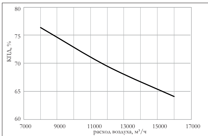
Температурный КПД теплоутилизатора
