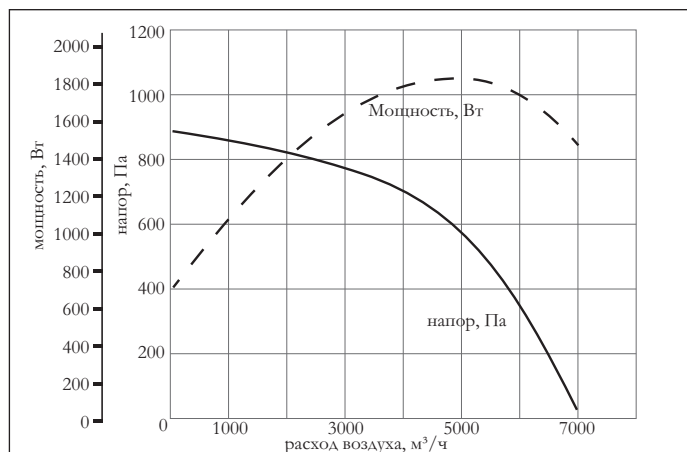
Аэродинамическая характеристика вентилятора
